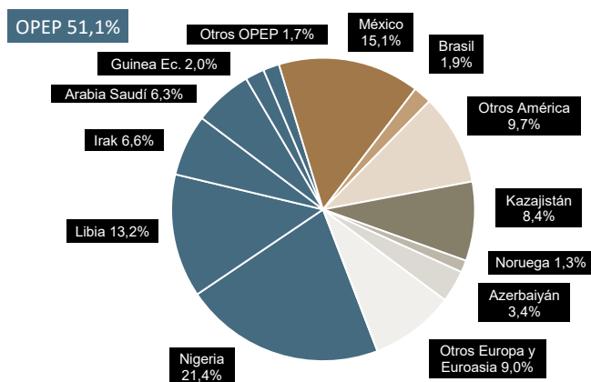
Distribución importaciones de crudo Enero-Marzo 2021
